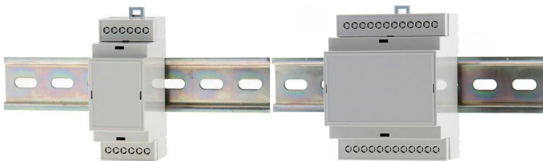
Рисунок 3.1 Внешний вид МРС-1ШП и МРС-1УП
