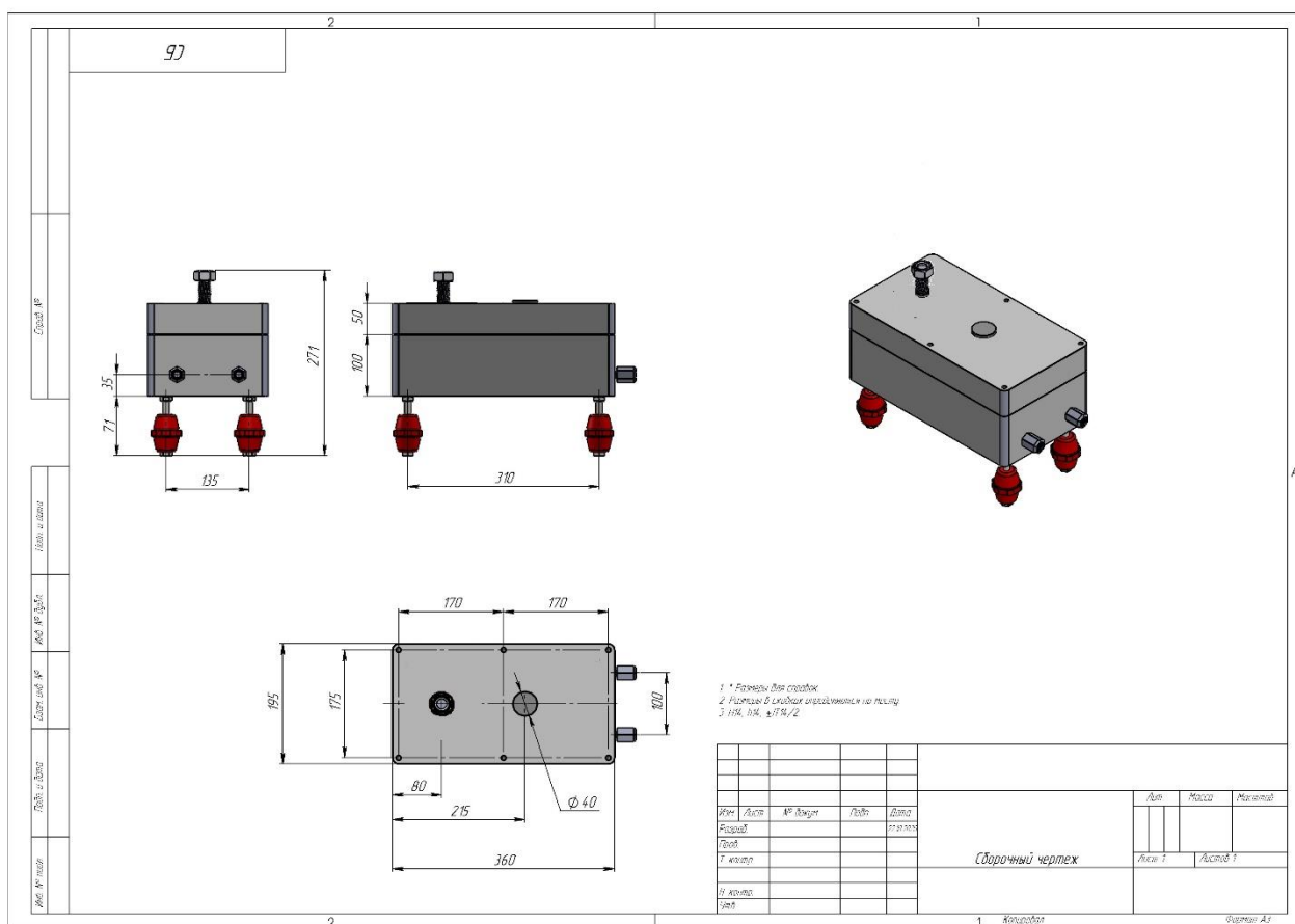
Рисунок 3.2 Чертеж Изделия
