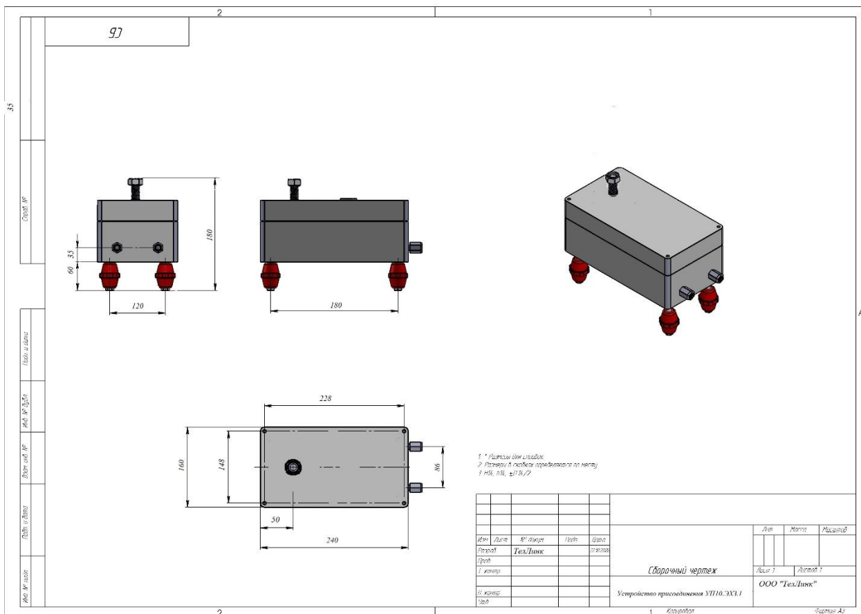
Рисунок 3.2 Чертеж Изделия
